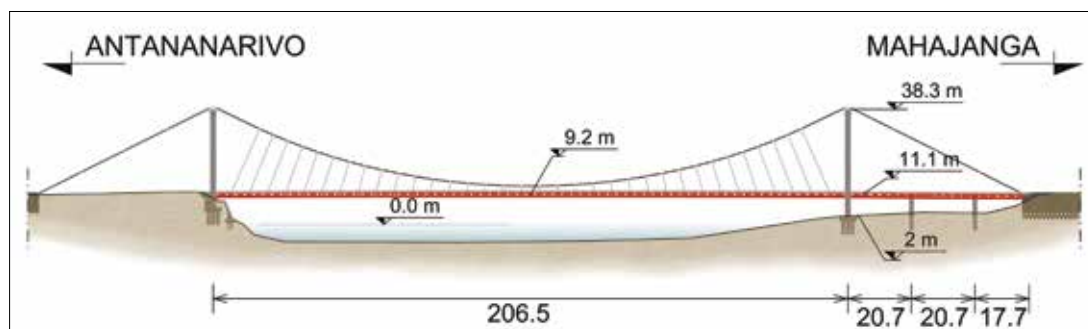
2. Il prospetto del nuovo ponte sospeso di Kamoro
